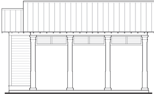
Right Elevation
